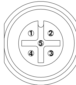
RS-232
